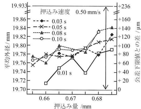
図6 平均外径に及ぼす押込み量と保持時間の影響
