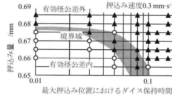
図5 M20×P1.5の中空ねじ転造の成形領域の例
