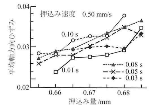
図8 軸方向伸びに及ぼす押込み量と保持時間の影響
