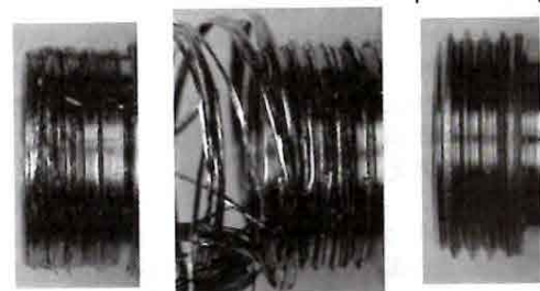
図4 押込み速度の違いにおけるねじ山の成形状況
