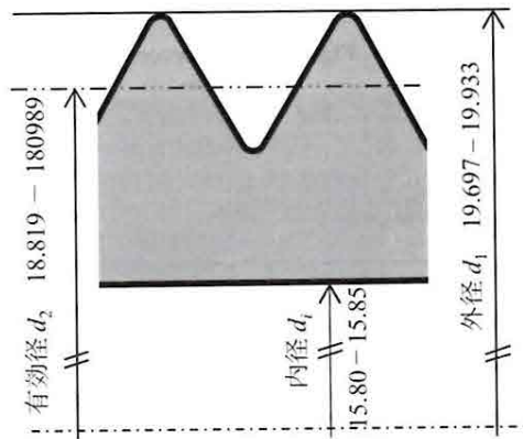
図3 実験した中空ねじの諸元 (M20×P1.5, 等級6e)
