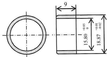
図2 素材の転造部
