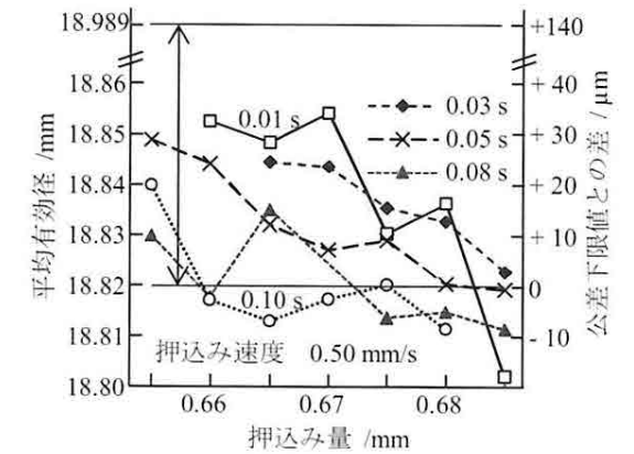
図7 平均有効径に及ぼす押込み量と保持時間の影響
